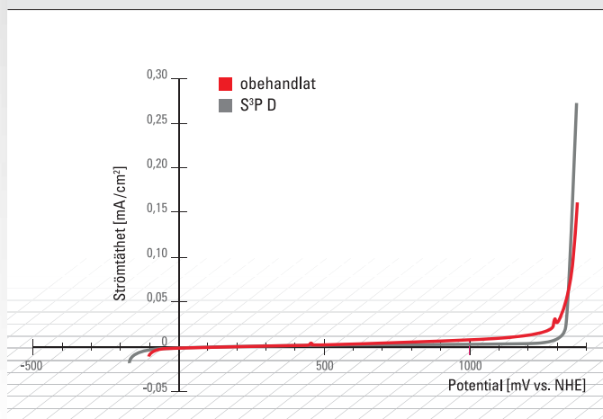
Summa-strömtäthet-potential-kurva för standardduplexstål 1.4462 i 3-procentig NaCl-lösning.
