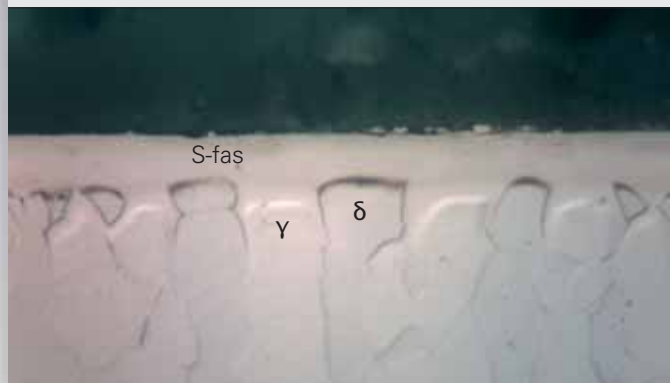
Strukturbild av ett S 3 P D-behandlat duplexstål 1.4462, bredare diffusionszon i den austenitiska fasen.
