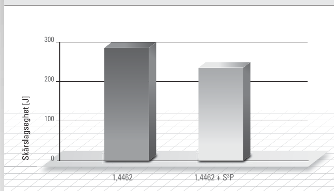
En lätt reduktion av skårslagsegheten hos material 1.4462 på grund av en partiell utskiljning av den ferritiska fasen.
